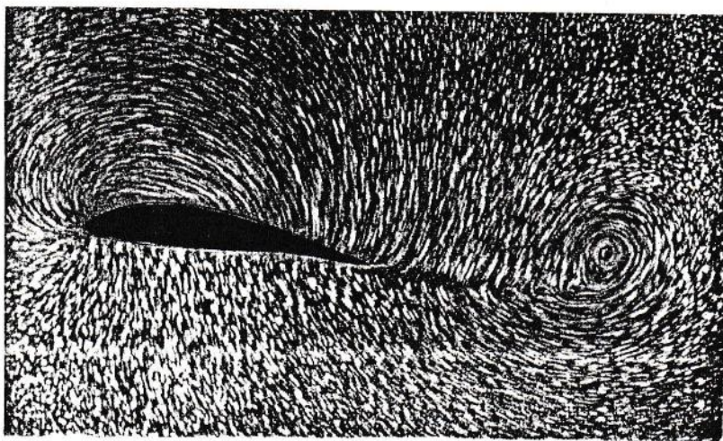
Corrente non stazionaria attorno ad un'ala, con vortice d'avviamento. La macchina fotografica trasla con velocità uguale alla velocità asintotica della corrente.
