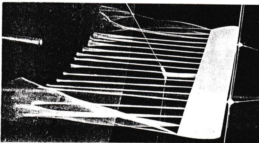
Visualizzazione con fili di lana della scia di Prandtl (nella galleria dell'Istituto di Aeronautica del Politecnico di Milano).
